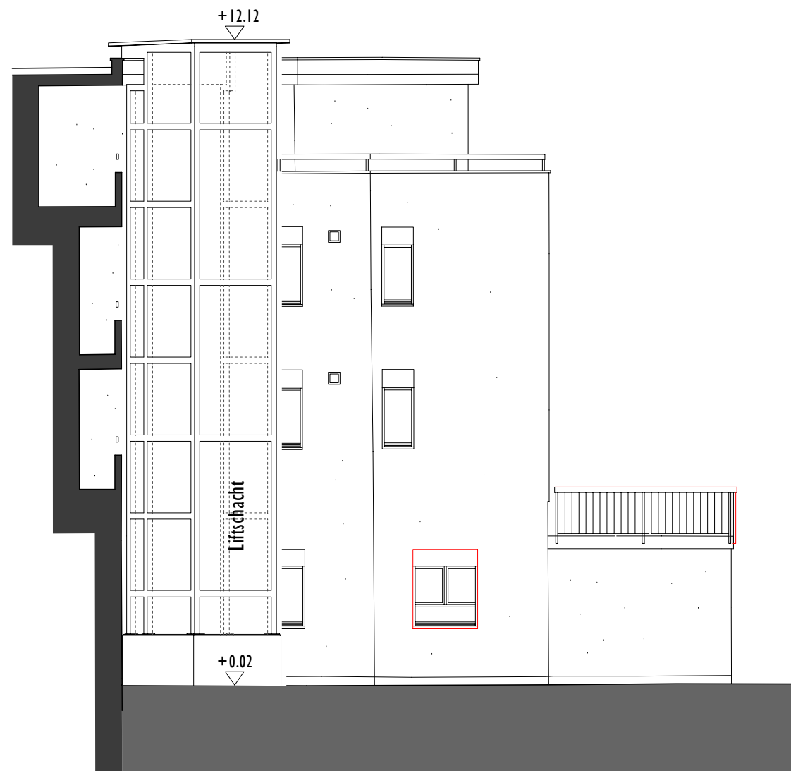
NORD-OSTFASSADE
